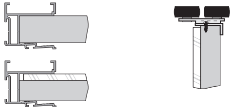
Способ монтажа угольника 11 мм. x 17 мм.
